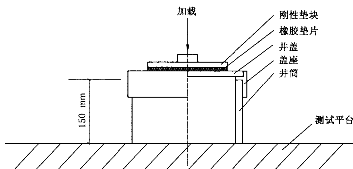
图 C.8 荷载试验
