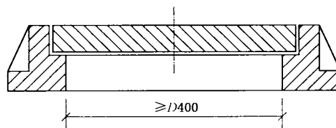
图 C.4 315 防护盖座控制尺寸图
