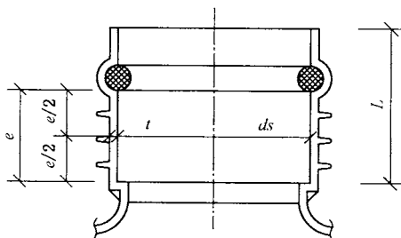
图 3 检查井井座与井筒连接部位带窝槽弹性密封承口示意图
